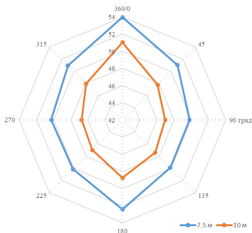
Рисунок 2. Диаграмма направленности легкового автомобиля на расстояниях 7.5 м и 10 м на холостом ходу
